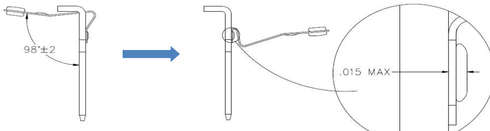
Figura 21 Dibujo de Remache
